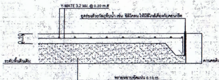
แบบขยายพื้น GS1
