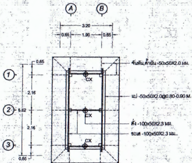
แบบแปลนหลังคากันสาด มาตราส่วน 1:100
