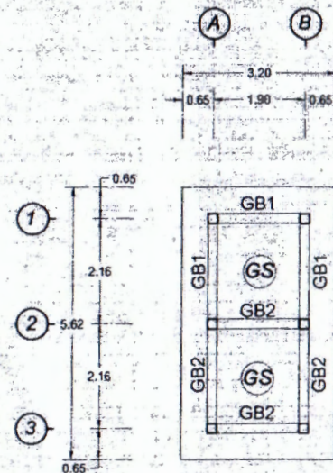
แบบแปลนคาน มาตราส่วน 1:100
