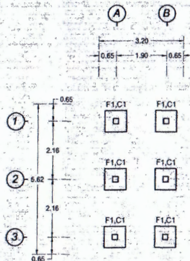
แบบแปลนฐานราก มาตราส่วน 1:100
