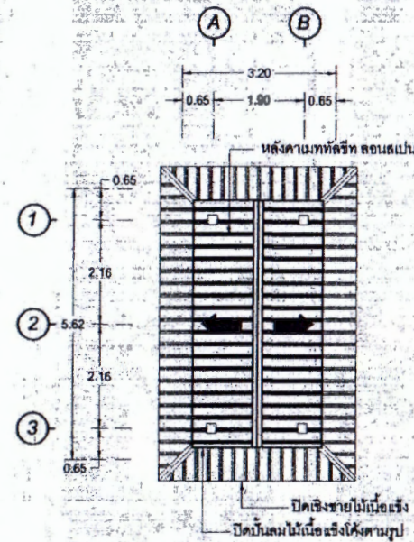
แบบแปลนหลังคา มาตราส่วน 1:100
