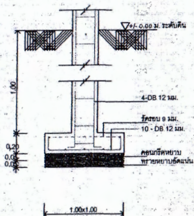
FOOTING F1 DETAIL SCALE 1:20
