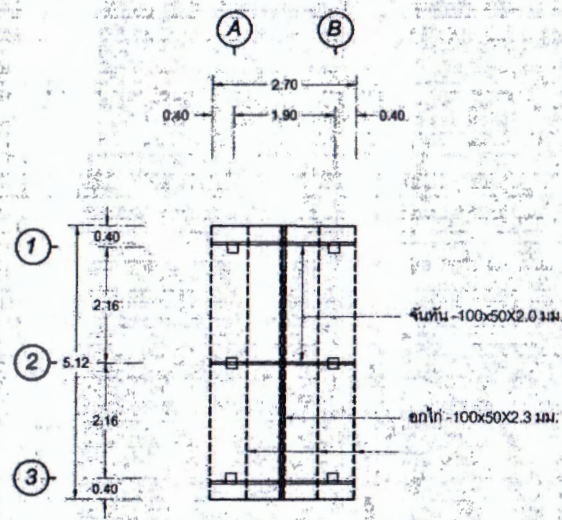
แบบแปลนหลังคาบน มาตราส่วน 1:100
